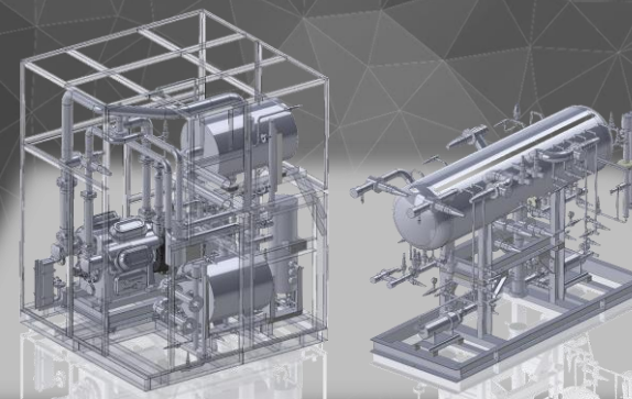
NH 3 /CO 2 冷却システム「NiCRES」
